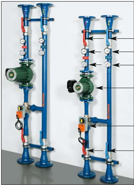
Regulación de calefacción 300 kW y 150 kW
