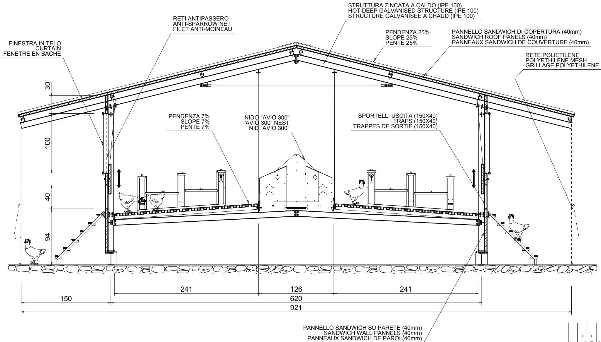
VISTA LATERALE TETTO ROOF SIDE VIEW VUE LATERAL DU TOIT
